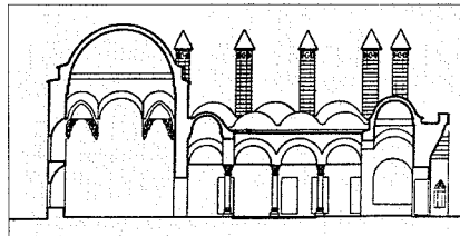
Gazi Hüsrev Bey Medresesi'nin planı ve kesiti
